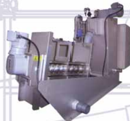
Déshydratation des boues à volute
